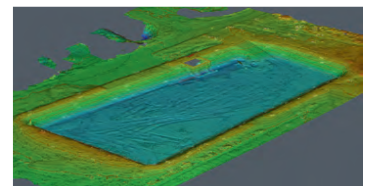
Orthophoto, digitales Geländemodell 2D- und 3D-Ansicht am Beispiel des Regenrückhaltebeckens Kevelaer
