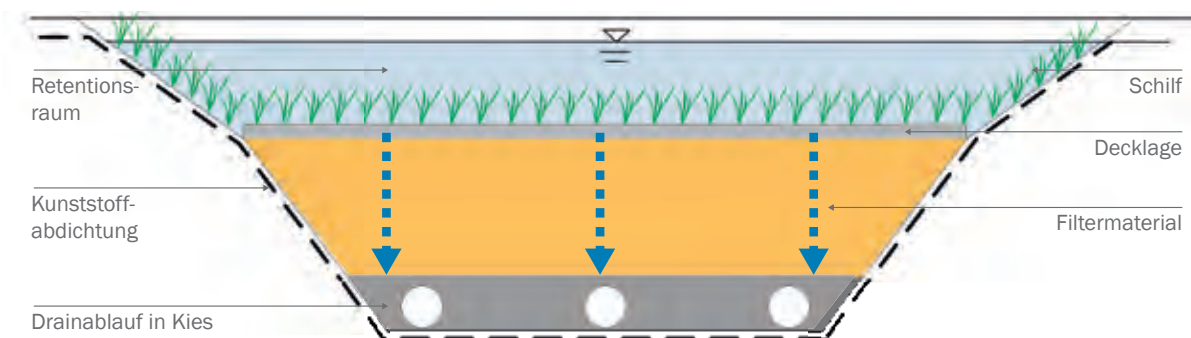
Schematischer Querschnitt eines Retentionsbodenfilters
